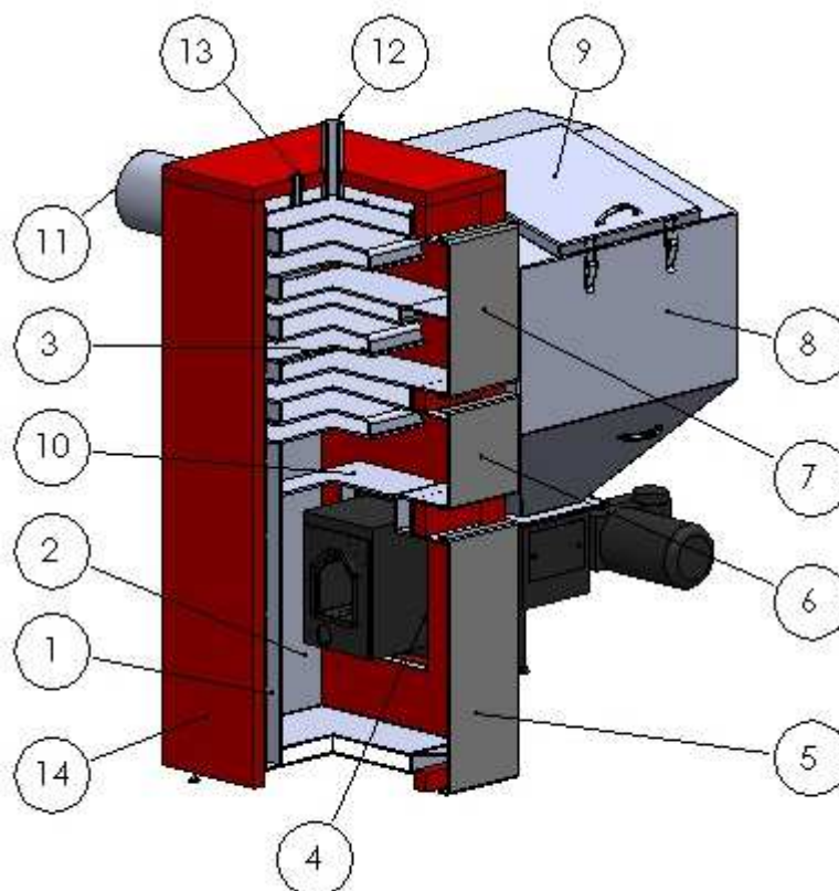
Rys.1. Kocioł "Technix (Uniwersal 5)"
