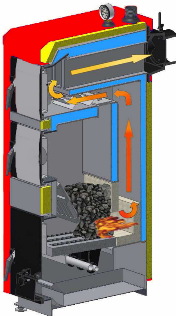
Obieg spalin w kotle UNIEKO
