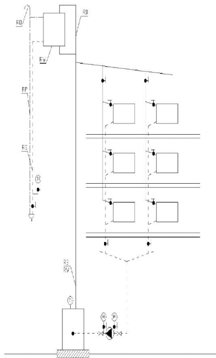
Rysunek 1b Schemat zabezpieczenia instalacji ogrzewania wodnego, wyposażonej w jeden kocioł lub wymiennik ciepła, rozdziel górną, pompą zamontowaną na powrocie wg PN-81/B-02413
