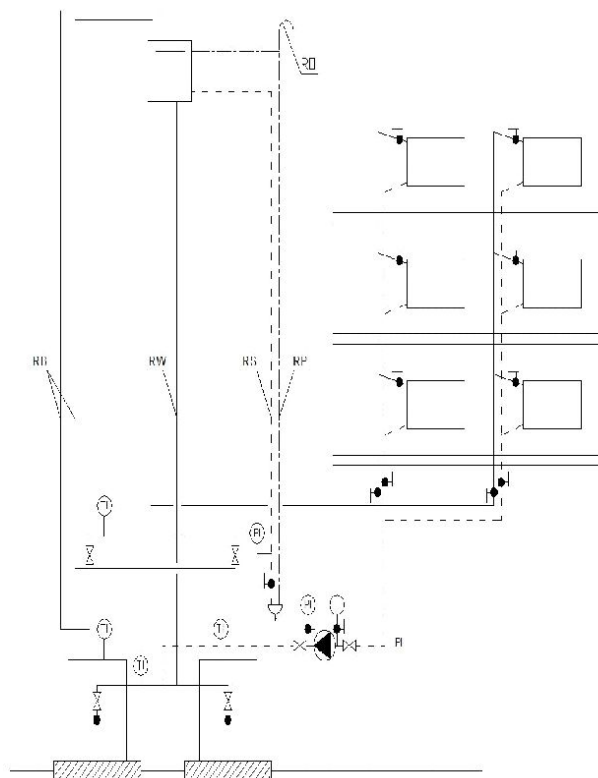
Rysunek 1c Schemat zabezpieczenia instalacji ogrzewania wodnego, wyposażonej w dwa lub więcej kotły lub wymienniki ciepła, rozdział górny, pompa zamontowana na powrocie wg PN-91/B-02413
