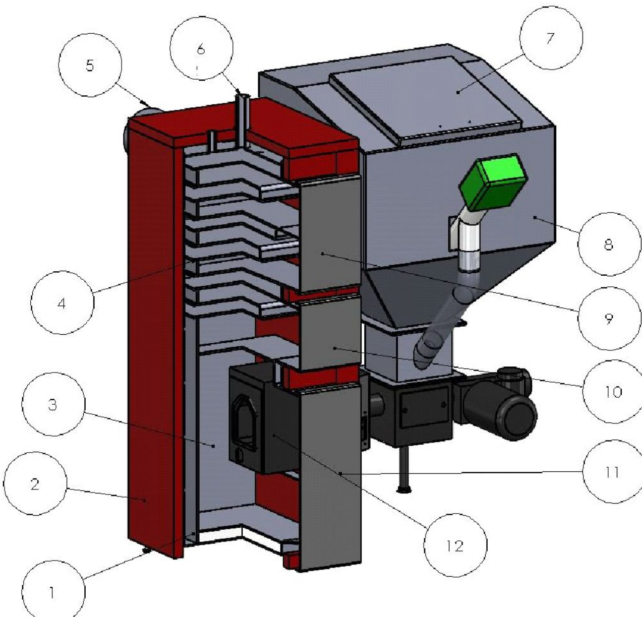
Rys.1. Kocioł "Technix-Pel"
