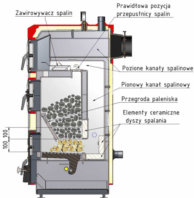
Sposób zasypu paliwa do kotła
